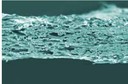
Struktur von Tyvek®: Durch den mehrschichtigen Aufbau aus Endlosfasern ist das Material unempfindlich gegen Abrieb und gibt weniger leicht Fusseln ab.
